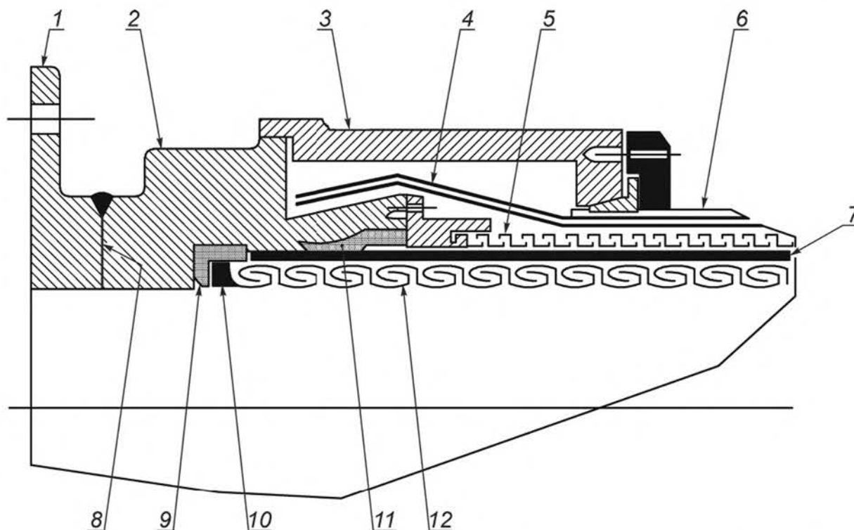
1 — монтажный фланец; 2 — корпус концевой фитинга (внутренняя оболочка); 3 — корпус концевой фитинга (наружная оболочка); 4 — армирующий слой, работающий на растяжение (залитый эпоксидным материалом); 5 — армирующий слой, обеспечивающий стойкость к давлению; 6 — наружная оболочка; 7 — внутренняя оболочка, работающая под давлением (и защитные слои); 8 — шейка концевой фитинга; 9 — торцевое уплотнение; 10 — замыкающее кольцо каркаса; 11 — радиальное уплотнение; 12 — каркас
