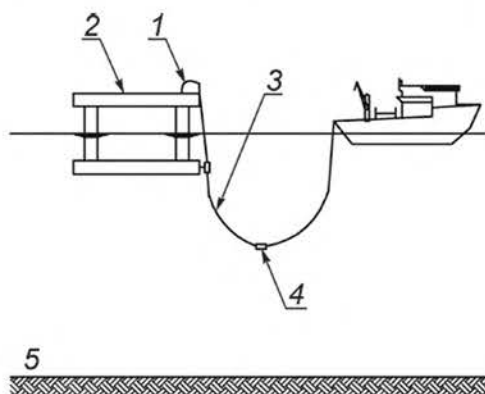
а) Втягивание REF
