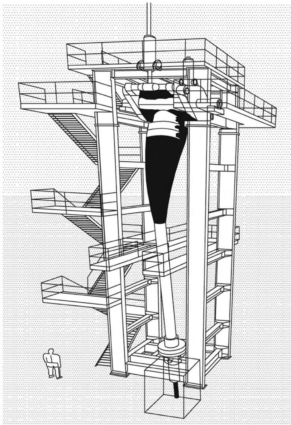
Рисунок 27 — Типовая установка для испытания на динамическую усталость
