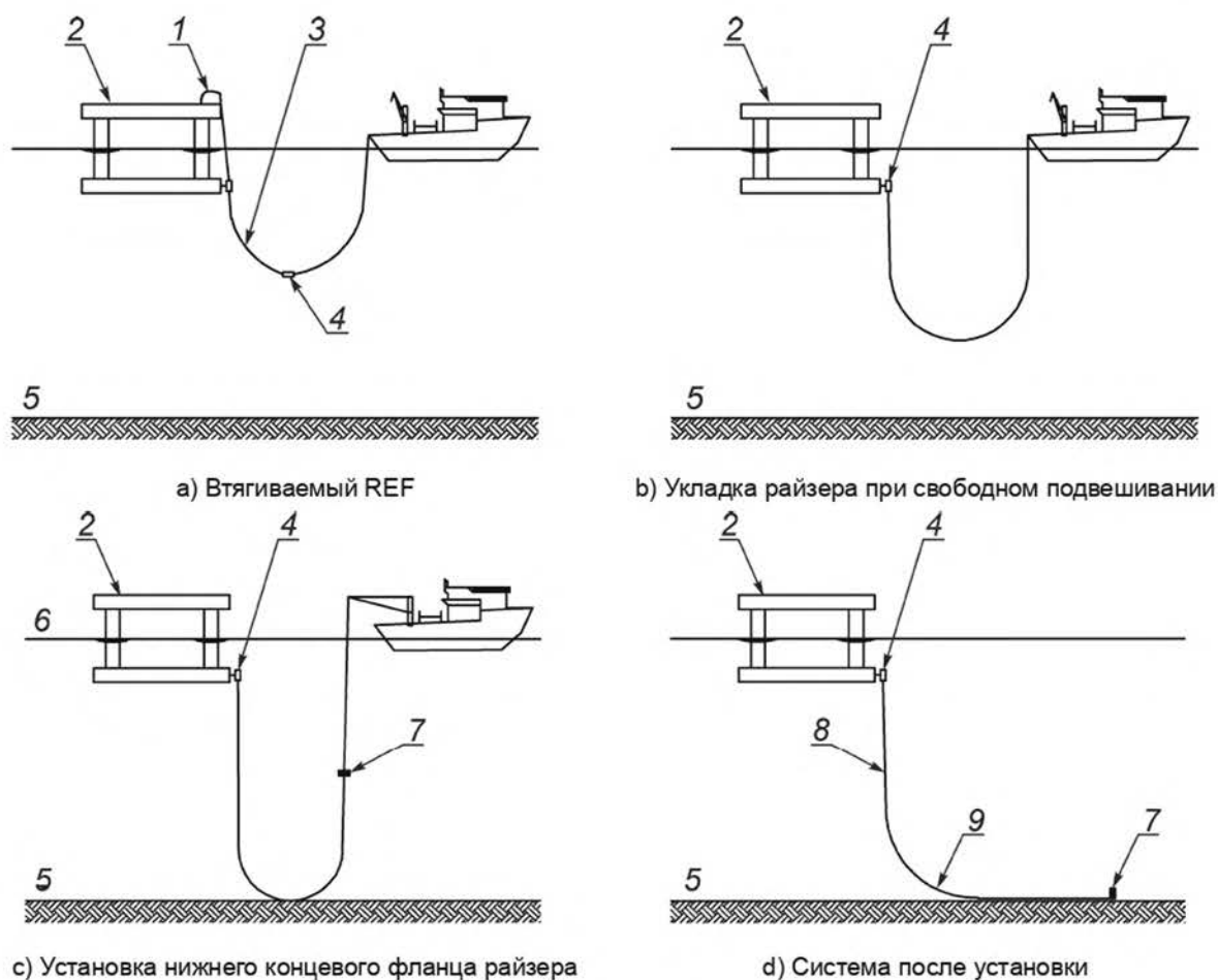
1 — втягивающая лебедка; 2 — FPS; 3 — втягивающий трос; 4 — REF; 5 — морское дно; 6 — средний уровень моря; 7 — фланец райзера; 8 — гибкий райзер; 9 — точка касания
