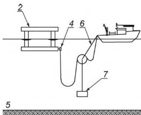
б) Установка подводного буя
