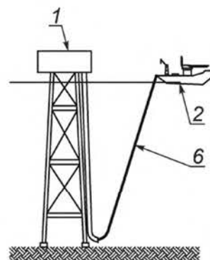
д) Достижение гибкой трубы верха J-образной трубы и прикрепление концевых фитингов к конструкции подвески
