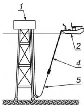
с) Втягивающий трос, прикрепляемый к концу гибкой трубы, и начало операции втягивания
