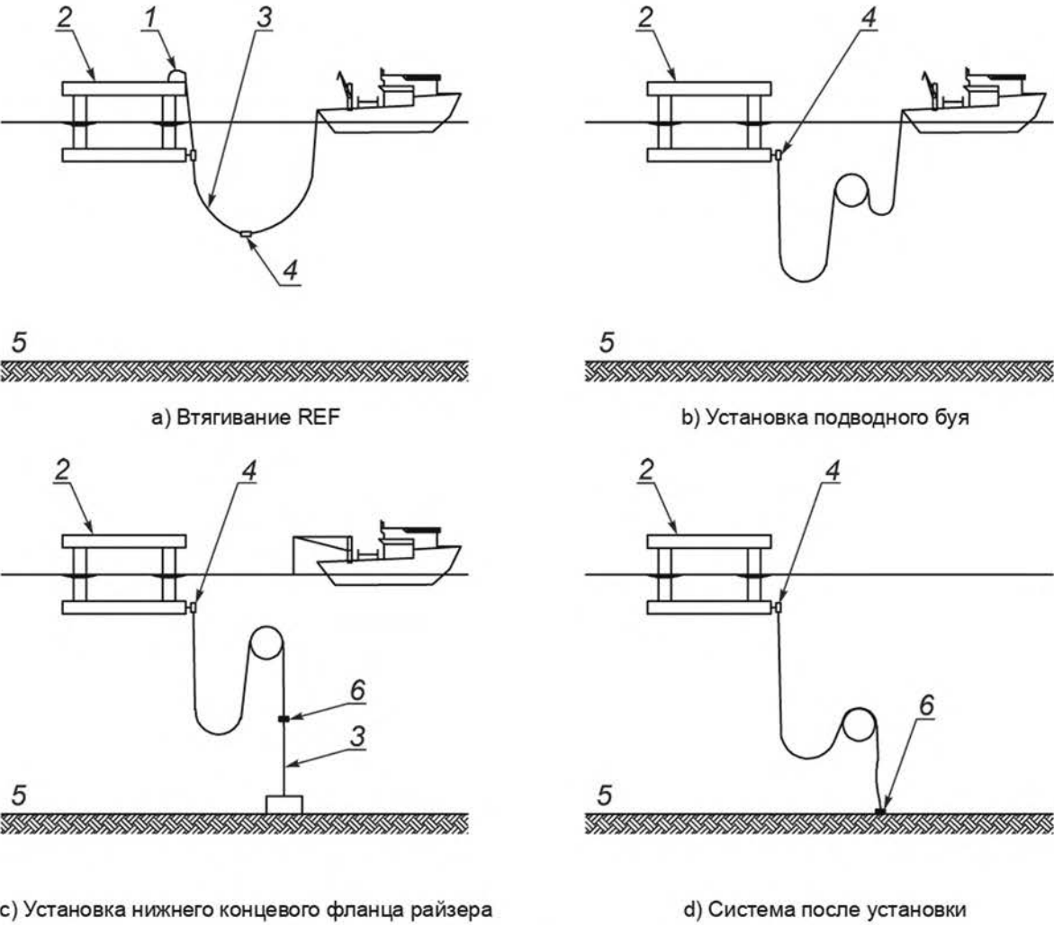
Рисунок 34 — Типовая процедура установки райзера в конфигурации крутого S-подъема
