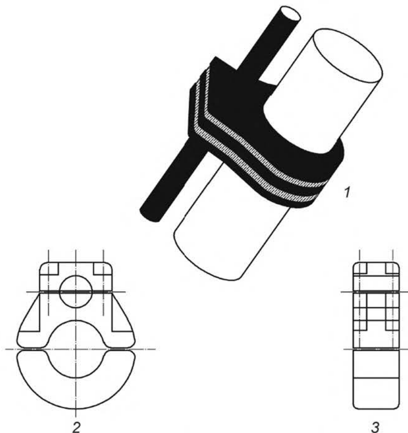
1 — хомут райзера; 2 — вид спереди; 3 — вид сбоку
