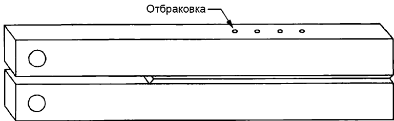
Рисунок D.30 — Расположение отпечатков при контроле твердости на образце DCB
