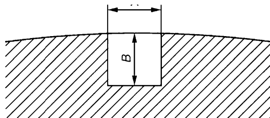
б) Надрез на наружной поверхности 3
