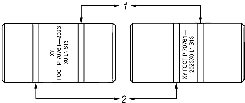
1 — полоса голубой краской на муфте с уплотнительными кольцами; 2— полоса(ы) для групп прочности или другие полосы Рисунок D.29 — Пример расположения полос в цветовой маркировке муфты с уплотнительными кольцами
