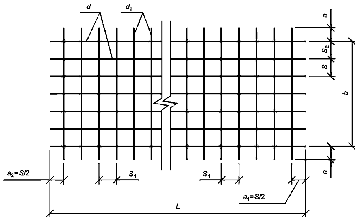
Рисунок 1 — Параметры сварной сетки
