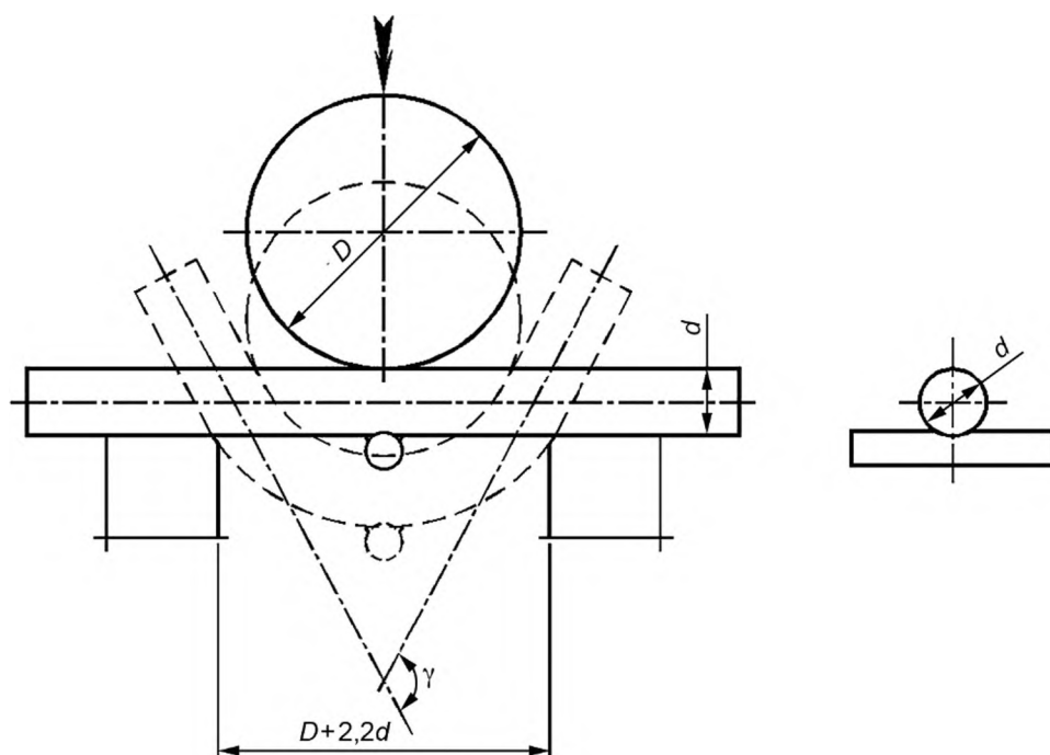
Рисунок Б.1 — Схема испытаний на изгиб крестообразных сварных соединений
